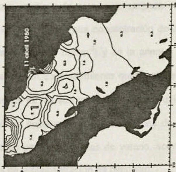
Figura 27.- Mapas de isolíneas de la concentración de pigmento derivada de las observaciones del CZCS en condiciones de invierno para los días 5, 6, 7, 10, 11 y 12 de abril de 1980.
