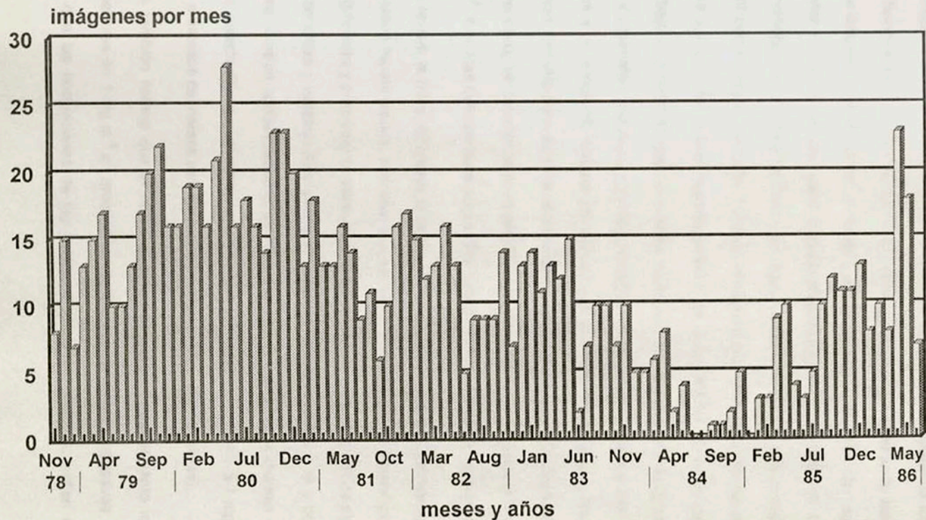
Figura 14.- Número de imágenes del CZCS, en composiciones diarias disponibles para el Golfo de California, en todo el período de la vida útil del CZCS.
