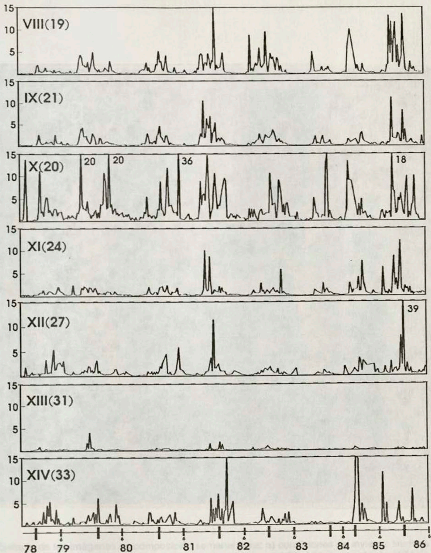
Figura 8.- Series de tiempo de la concentración de pigmento en promedios semanales para las regiones de la VIII a la XIV ejemplificadas por las localidades 19, 21, 20, 24, 27, 31 y 33 respectivamente. Las concentraciones de pigmento abarcan los años de 1978 a 1986, los números cerca de los picos son las concentraciones máximas alcanzadas por los mismos. Las concentraciones están expresadas \text{mg m}^3 .
