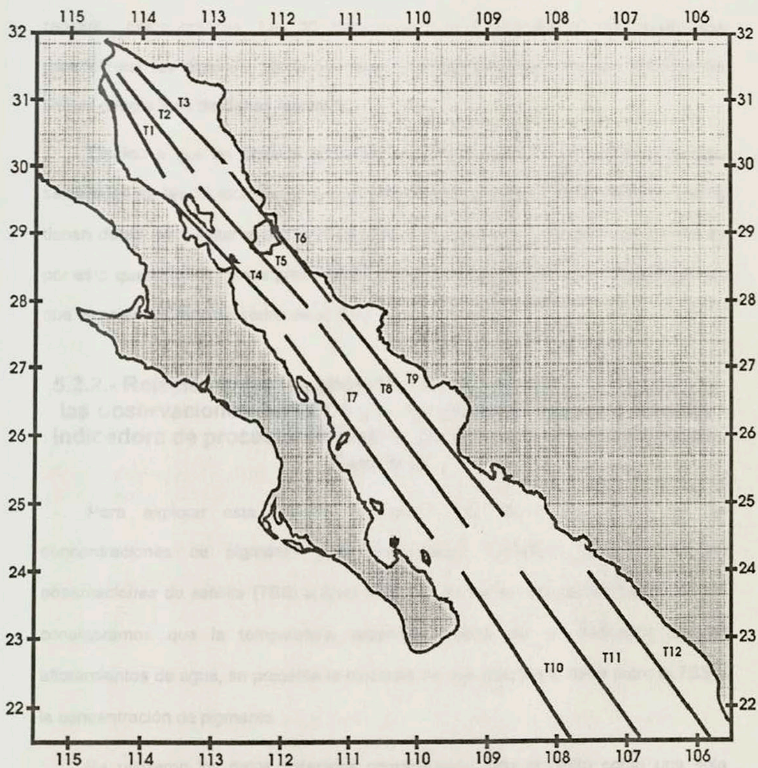
Figura 5.- Localización geográfica de los 12 transectos.
