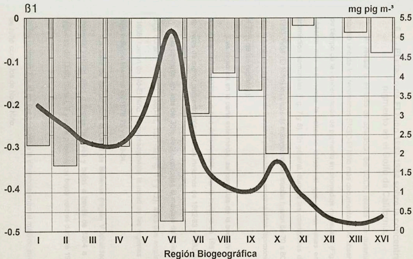
Figura 10.- Relación de la concentración de pigmento (línea) y el coeficiente \beta_1 (barras) por región biogeográfica.
