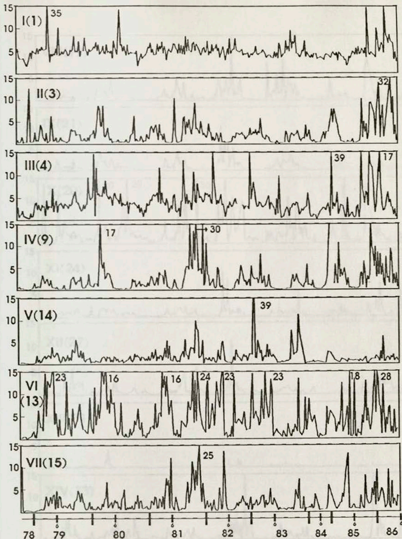
Figura 7.- Series de tiempo de la concentración de pigmento en promedios semanales para las regiones biogeográficas I, II, III, IV, V, VI y VII ejemplificadas por las localidades; 1, 3, 4, 9, 14, 13 y 15 respectivamente. Las concentraciones de pigmento abarca los años de 1978 a 1986, los números cerca de los picos son las concentraciones máximas alcanzadas por los mismos. Las concentraciones están expresadas en \text{mg m}^{-3} .
