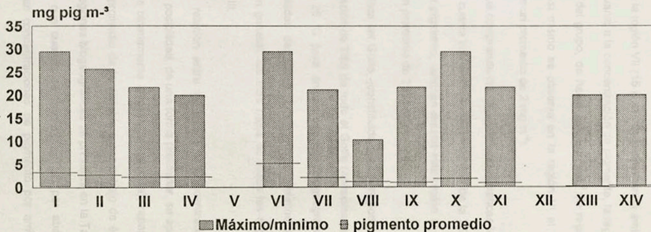
Figura 9.- Máximos/mínimos y promedios por región biogeográfica para el periodo de mayo de 1983 a junio de 1986; a) Temperaturas superficiales derivadas de las observaciones del AVHRR, expresadas en °C (TSS); b) Concentraciones de pigmento derivadas de las observaciones del CZCS, expresadas en mg m -3 .
